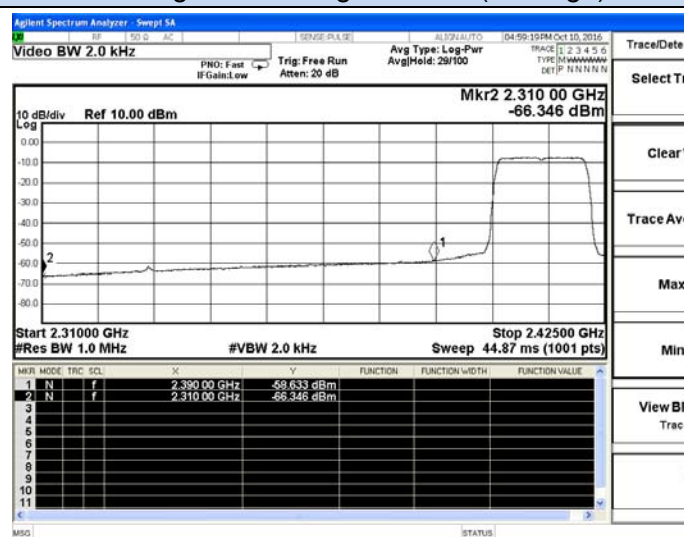
802.11n-HT20 Chain 0-Low channel(Average)
