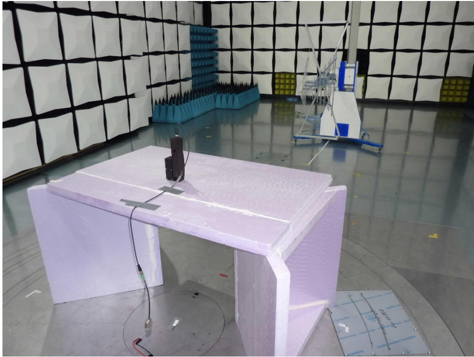
191513AS_03:Final Mesurement 30 – 1000 MHz
