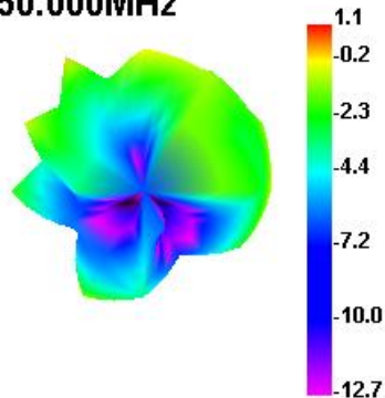
5650.000MHz E1
