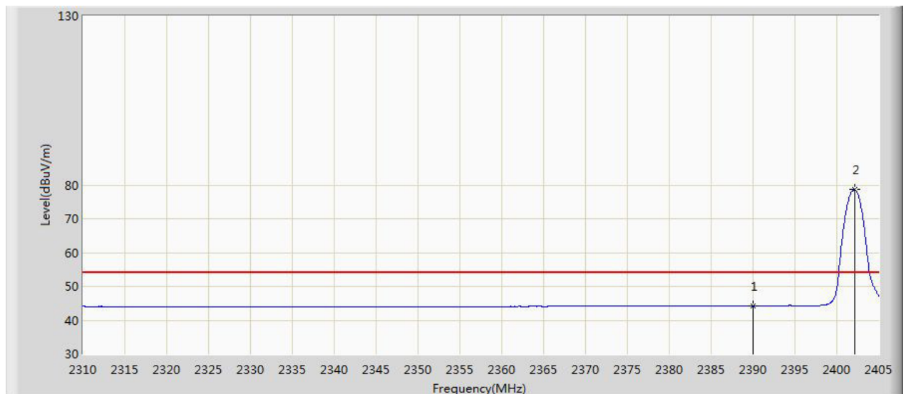
Figure 44: Band Edge, 3-DH5, 2402MHz, Vertical, AV
