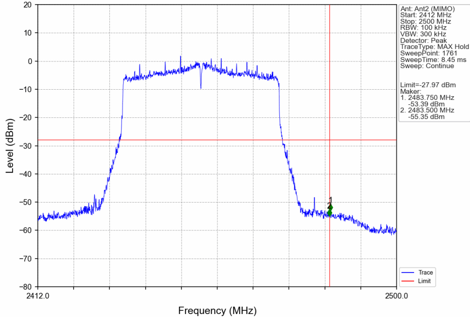
802.11ax(HEW40)_HCH_2452MHz_RU484_Left_Ant2 (MIMO)_NTNV
