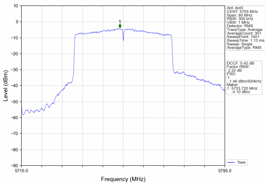
802.11ax(HEW40)_LCH_5755MHz_RU484_Left_Ant3_NTNV
