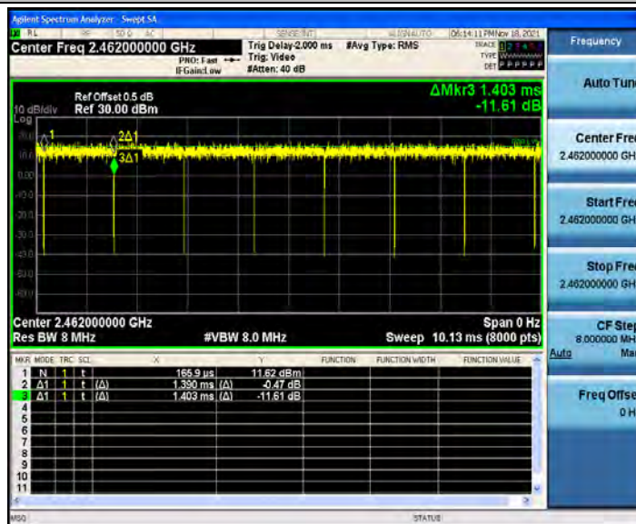
802.11g_Ant2_2462
