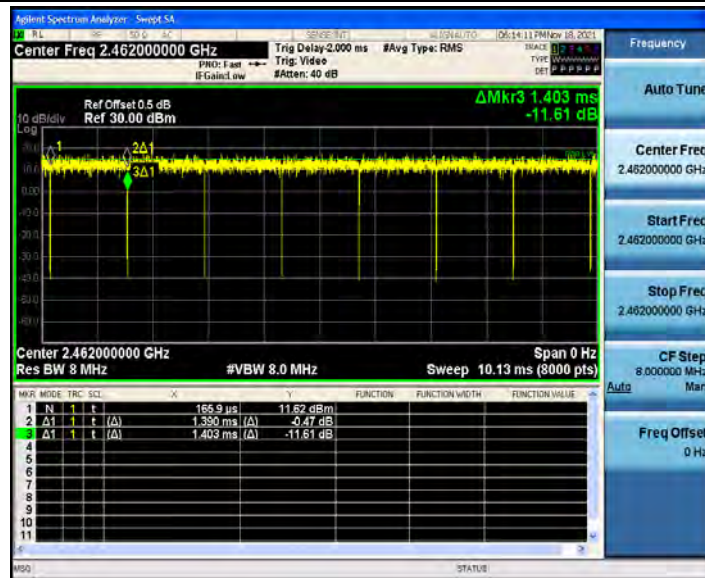
802.11g_Ant2_2462
