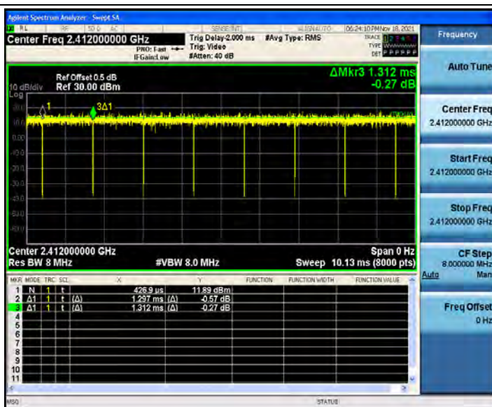
802.11n(HT20)_Ant2_2412
