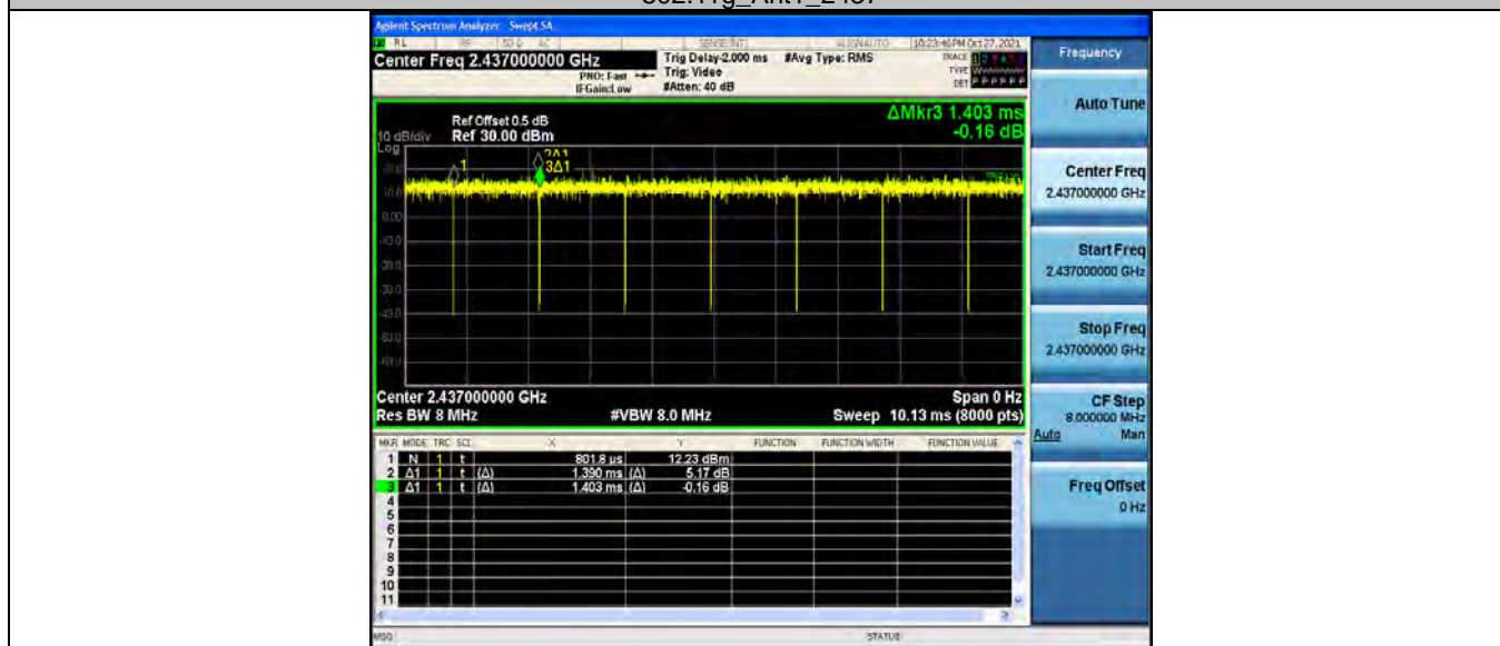
802.11g_Ant2_2437
