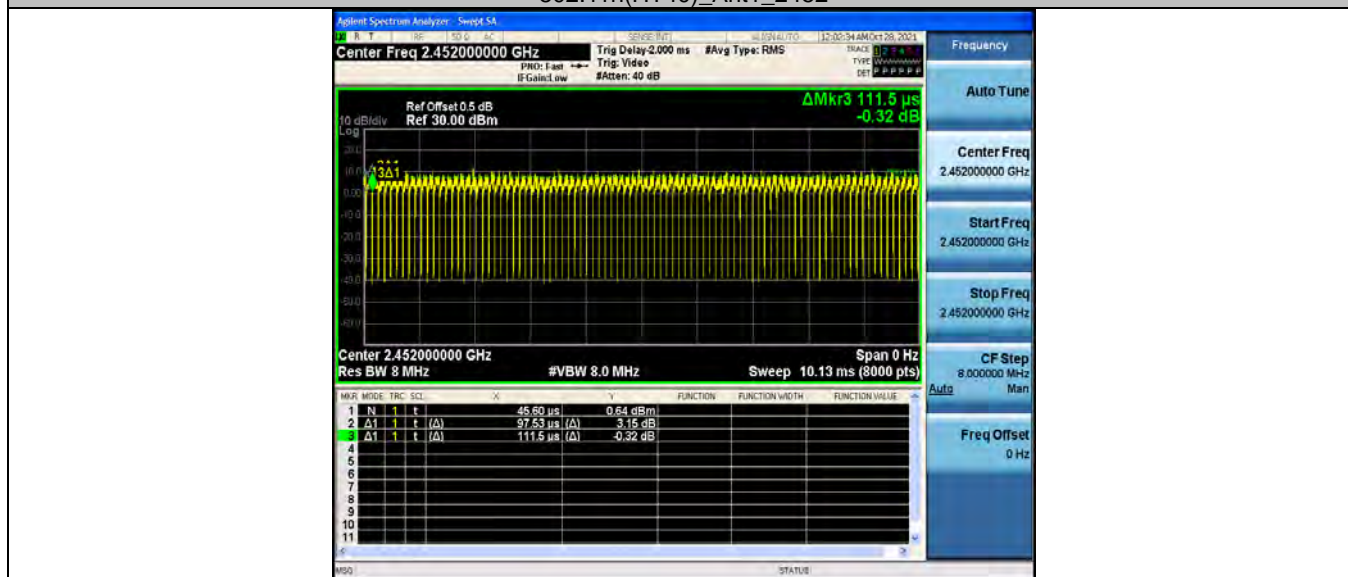
802.11n(HT40)_Ant2_2452
