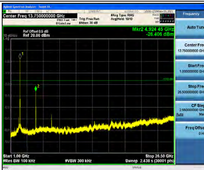
802.11b_Ant2_2462_0~Reference
