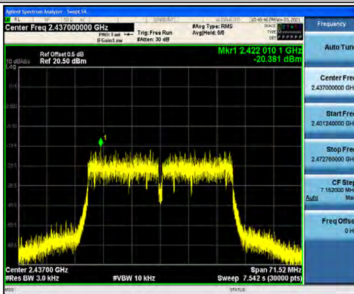
802.11n(HT40)_Ant2_2437
