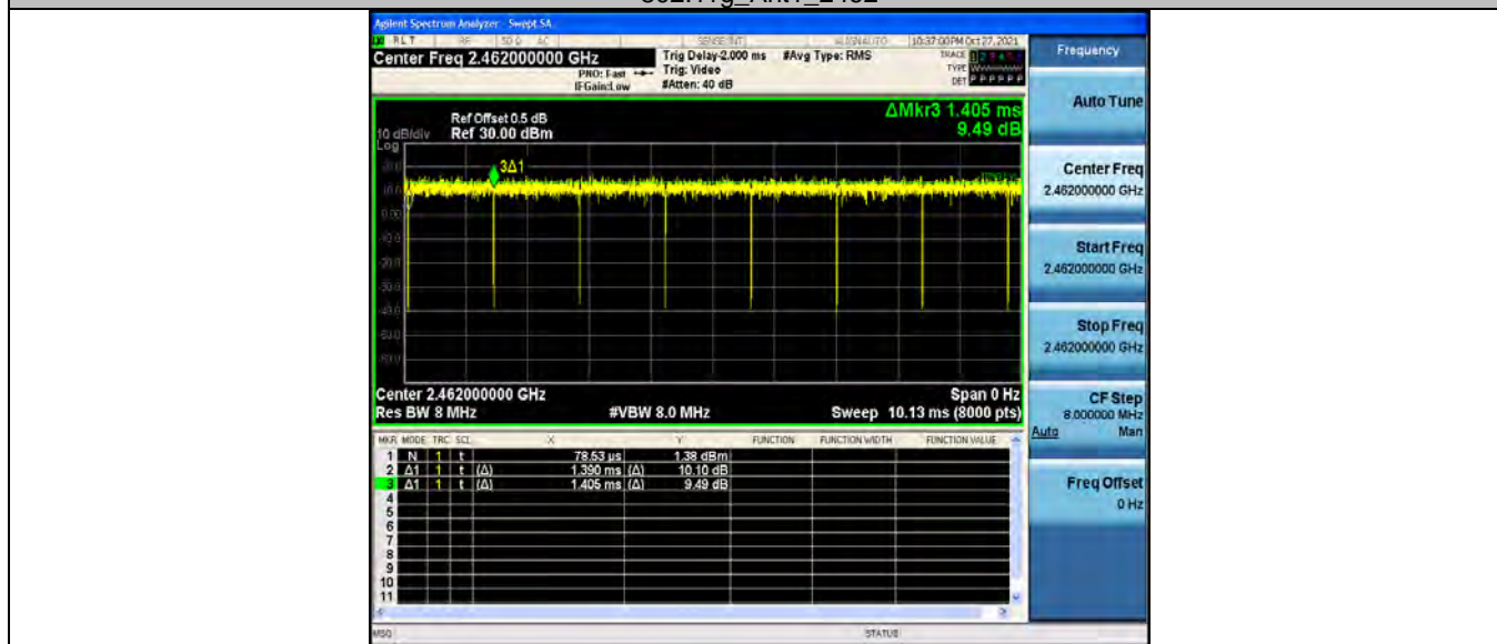
802.11g_Ant2_2462
