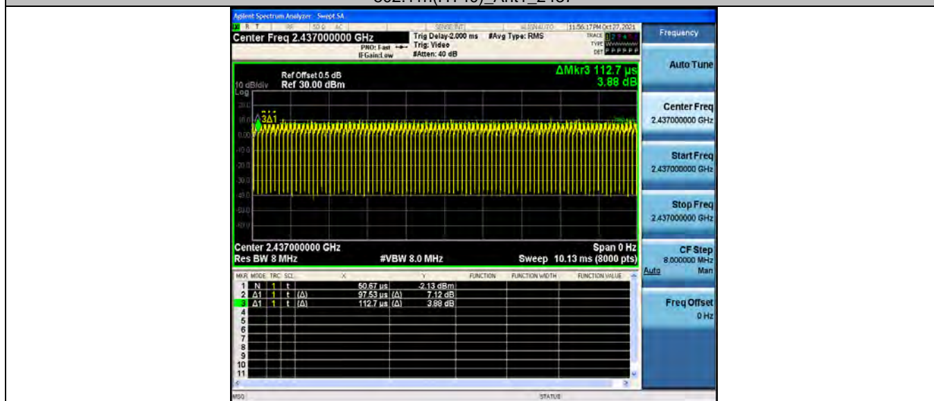
802.11n(HT40)_Ant2_2437
