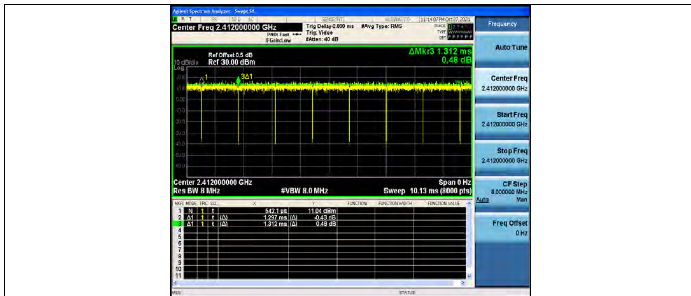
802.11n(HT20)_Ant2_2412
