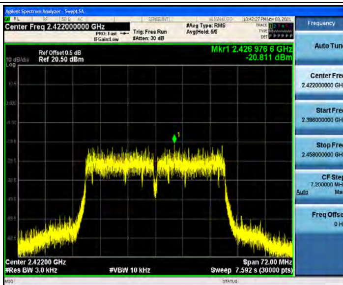
802.11n(HT40)_Ant2_2422
