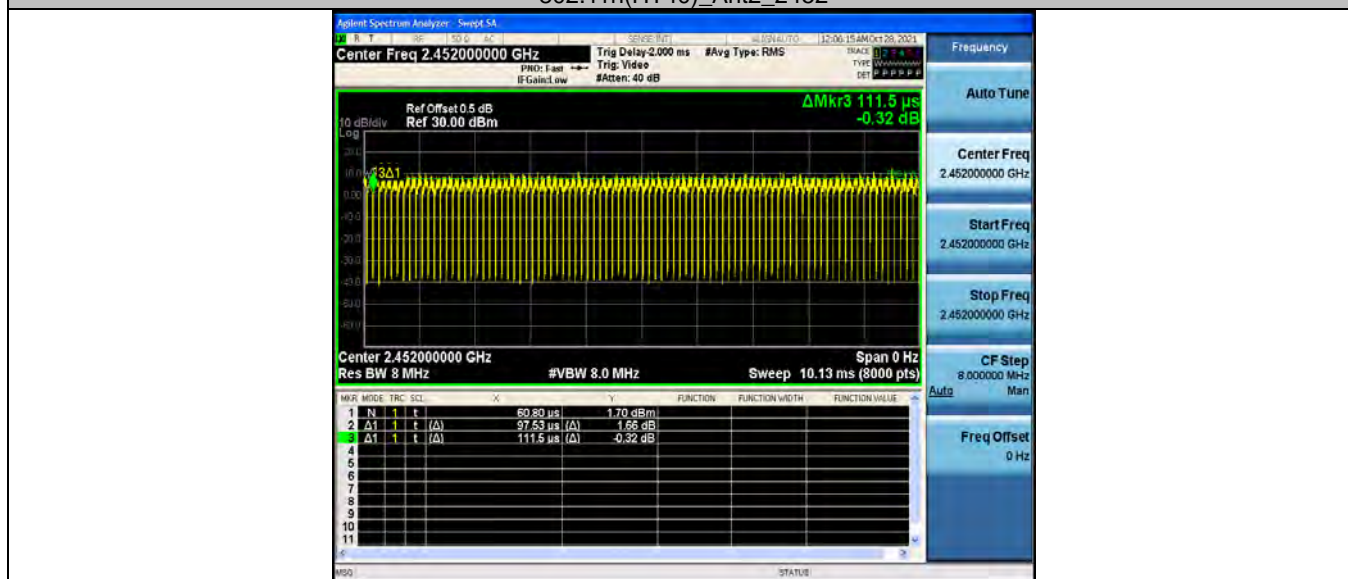
802.11n(HT40)_Ant2_2452
