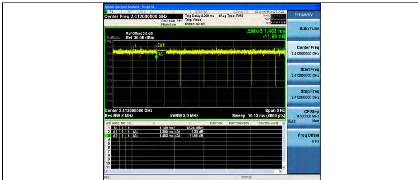
802.11g_Ant2_2412
