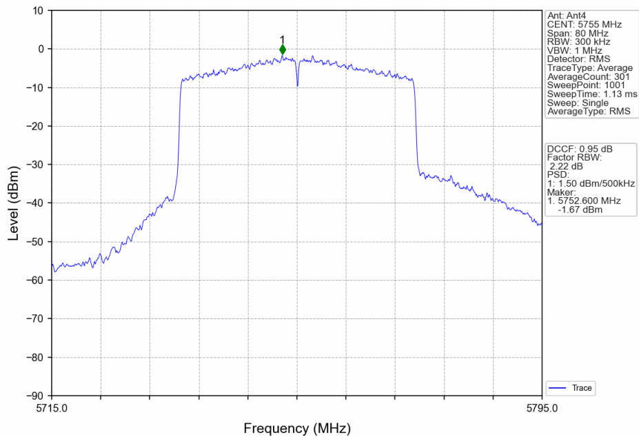
802.11ax(HEW40)_LCH_5755MHz_RU484_Left_Ant4_NTNV
