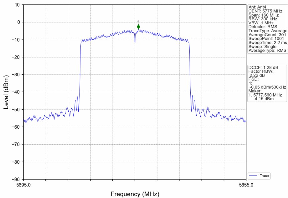
802.11ax(HEW80)_MCH_5775MHz_RU996_Left_Ant4_NTNV
