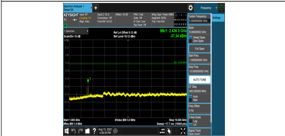
Band13-5MHz-QPSK-23230-1RB#0-Range4:1000~10000MHz
