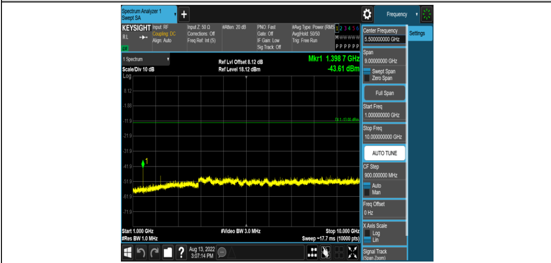
Band12-1.4MHz-QPSK-23017-1RB#0-Range4:1000~10000MHz
