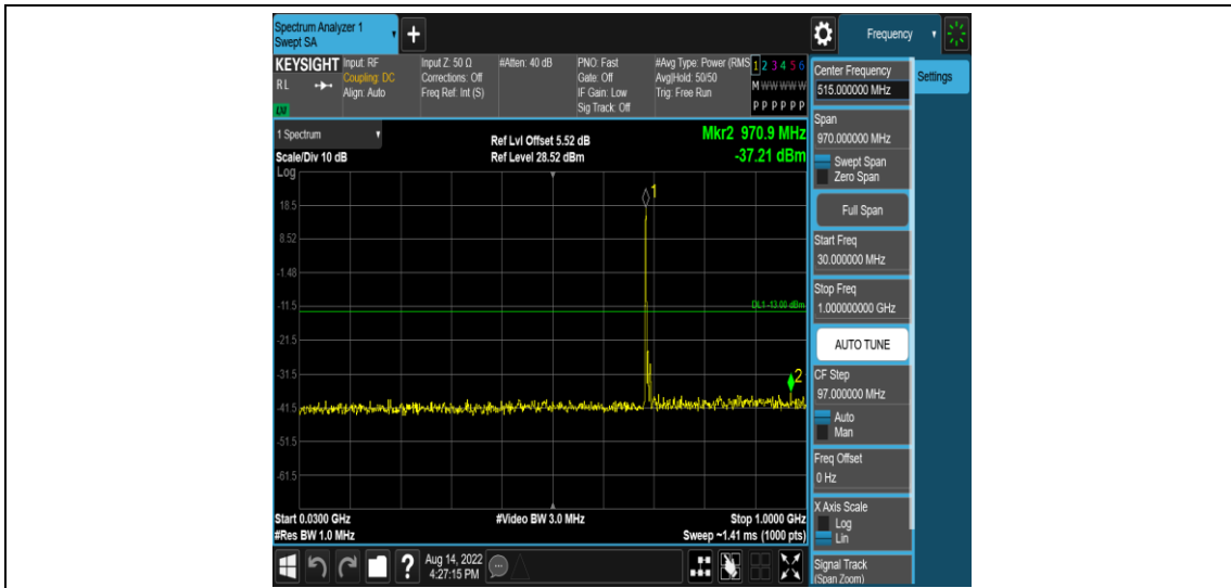
Band71-5MHz-QPSK-133447-1RB#0-Range3:30~1000MHz
