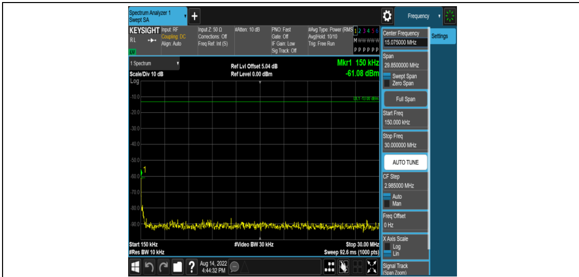
Band71-10MHz-QPSK-133172-1RB#0-Range2:0.15~30MHz
