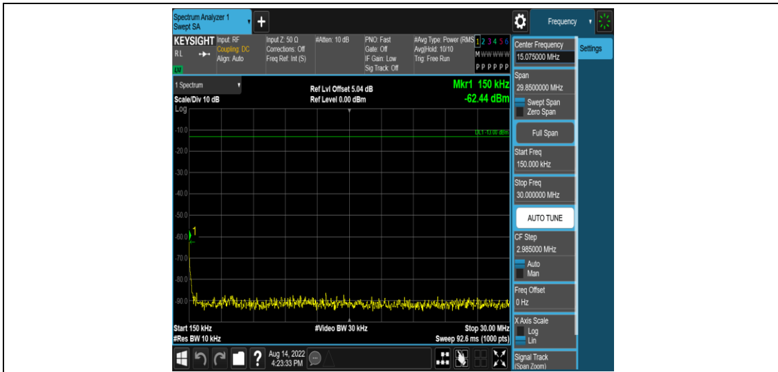
Band71-5MHz-QPSK-133147-1RB#0-Range2:0.15~30MHz
