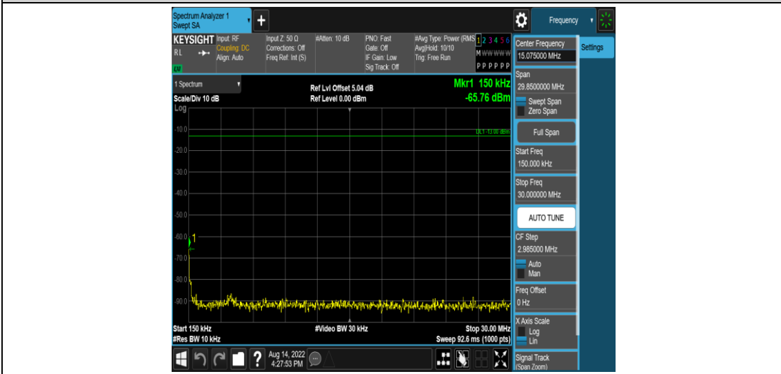
Band71-5MHz-16QAM-133447-1RB#0-Range2:0.15~30MHz
