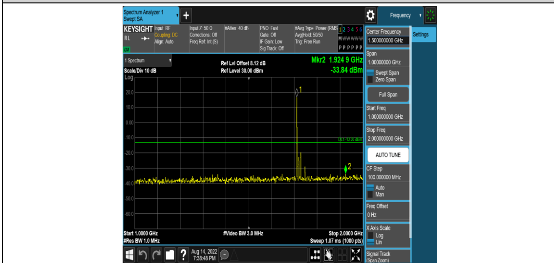
Band4-20MHz-QPSK-20050-1RB#0-Range4:1000~2000MHz
