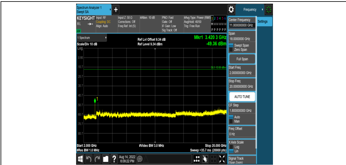
Band4-3MHz-QPSK-19965-1RB#0-Range5:2000~20000MHz
