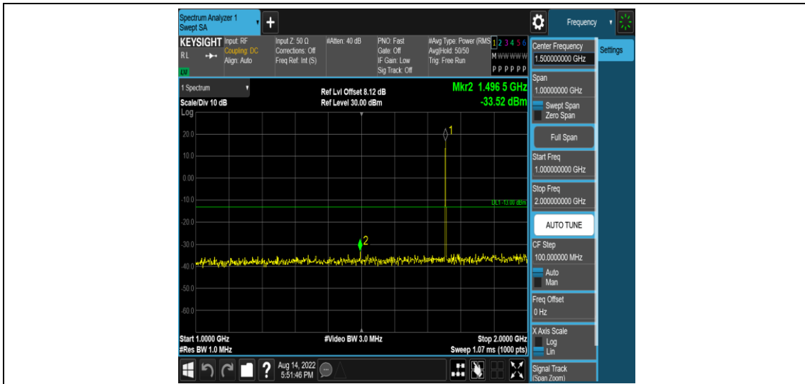
Band4-1.4MHz-QPSK-20393-1RB#0-Range4:1000~2000MHz
