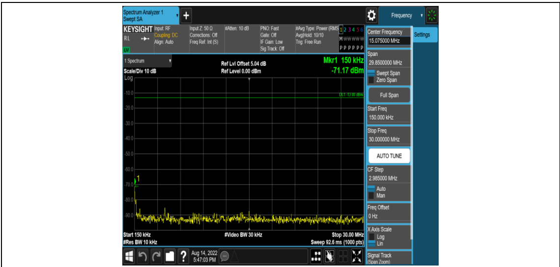
Band4-1.4MHz-QPSK-19957-1RB#0-Range2:0.15~30MHz
