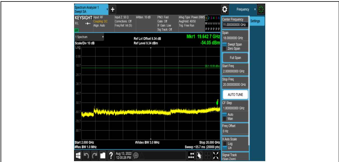
Band2-20MHz-QPSK-18700-1RB#0-Range5:2000~20000MHz
