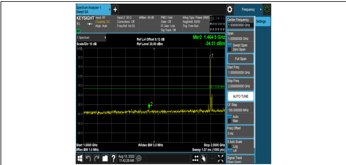
Band2-15MHz-QPSK-19125-1RB#0-Range4:1000~2000MHz
