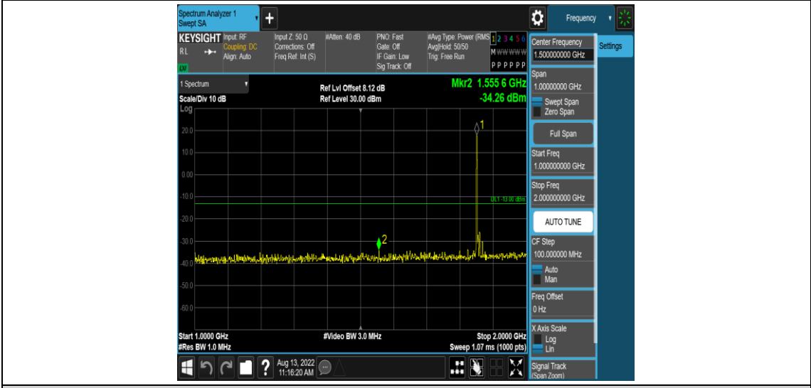
Band2-10MHz-QPSK-18650-1RB#0-Range4:1000~2000MHz
