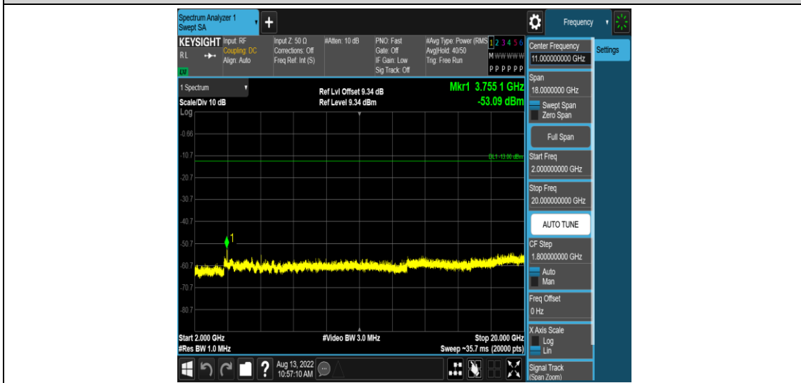
Band2-5MHz-QPSK-18900-1RB#0-Range5:2000~20000MHz
