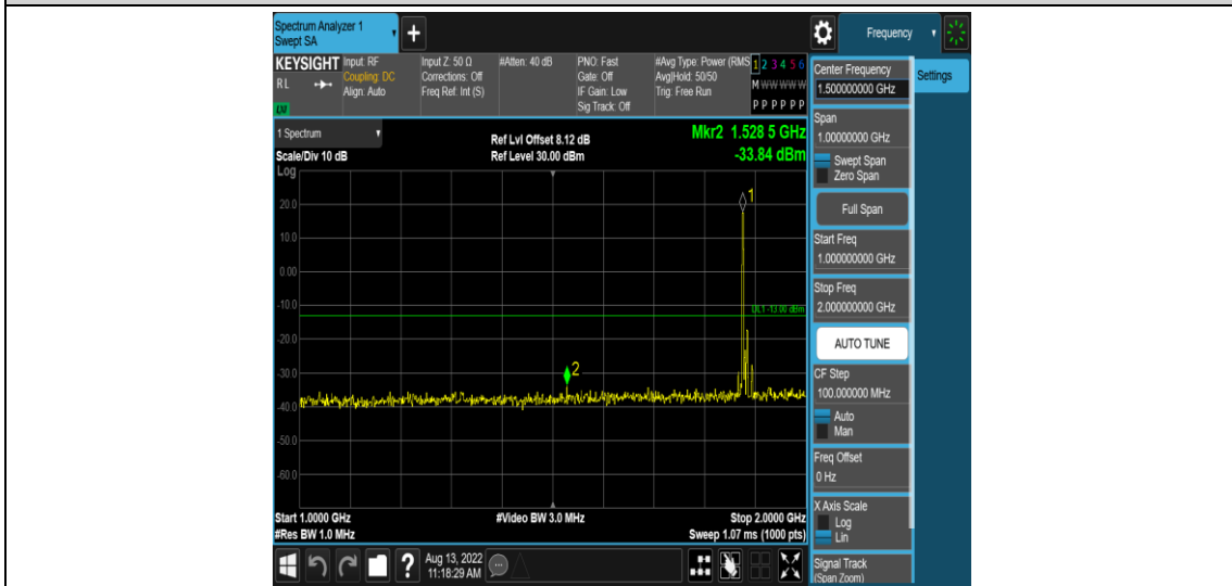
Band2-10MHz-QPSK-18900-1RB#0-Range4:1000~2000MHz
