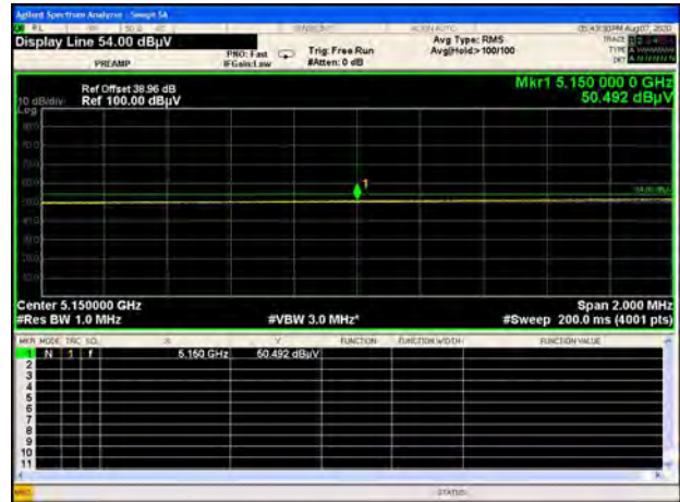
U-NII-1 11a CH36 AV
