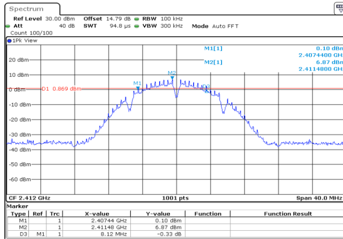
11bMIMO_Ant1_2412
