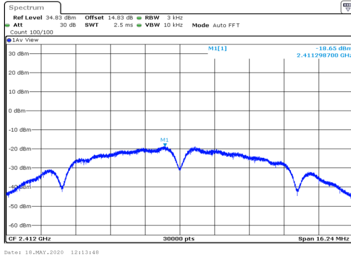
11bMIMO_Ant2_2412
