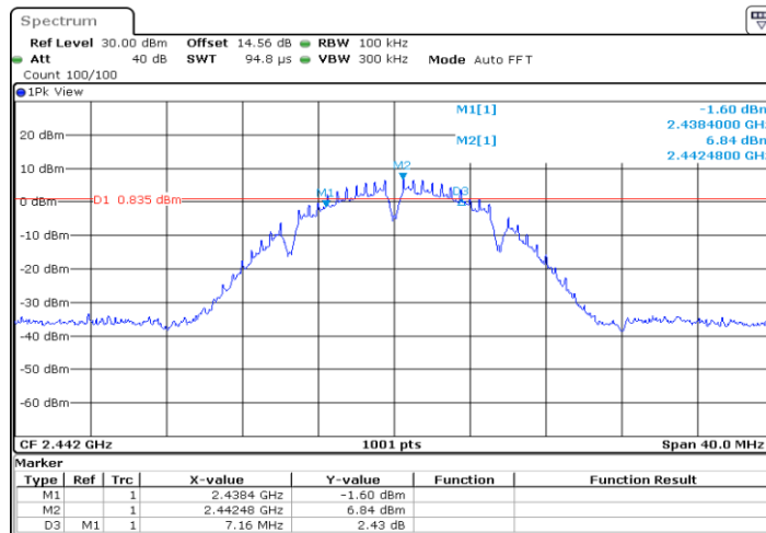
11bMIMO_Ant1_2442
