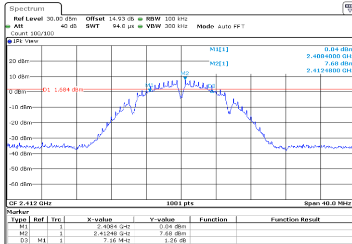
11bMIMO_Ant2_2412
