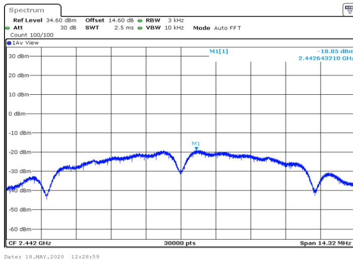
11bMIMO_Ant1_2442
