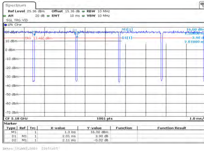
11A-MIMO_Ant2_5180
