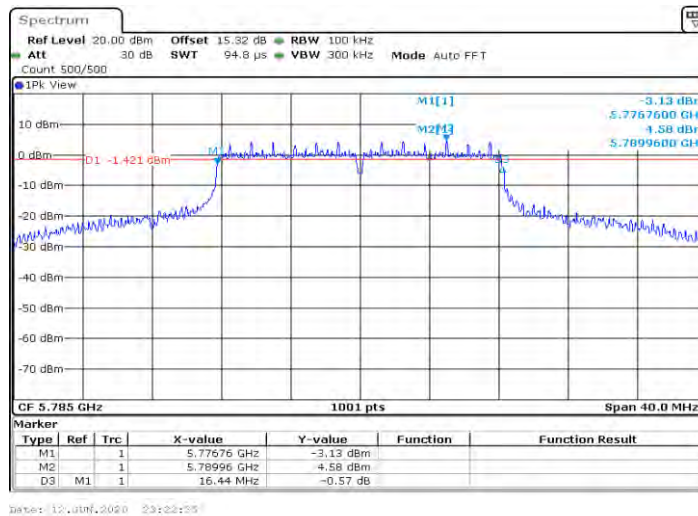
11A-MIMO_Ant1_5785
