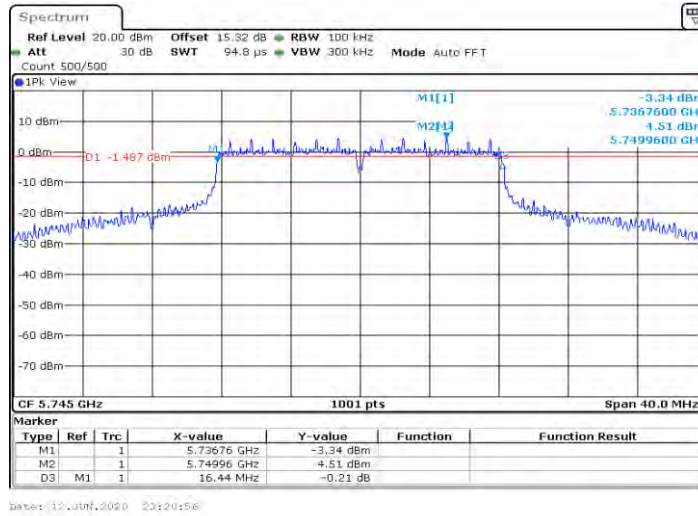
11A-MIMO_Ant2_5745
