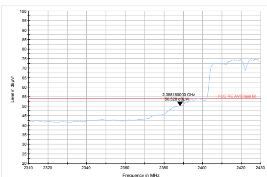
802.11n(HT40), Channel No. 3 - AV
