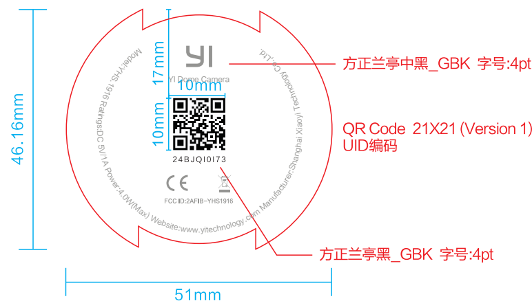
尺寸标示图:
