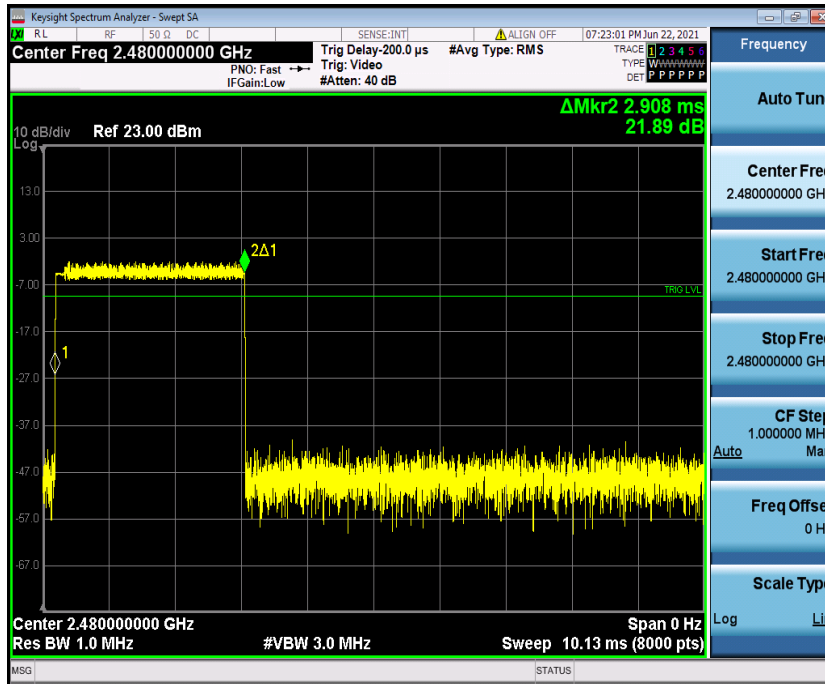
3DH5_Ant1_Hop_2480
