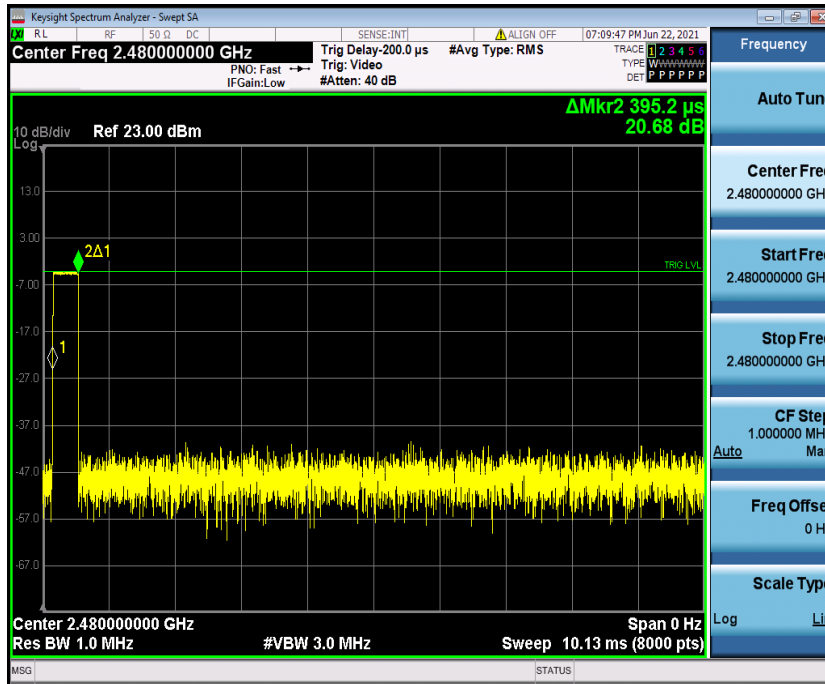
DH1_Ant1_Hop_2480
