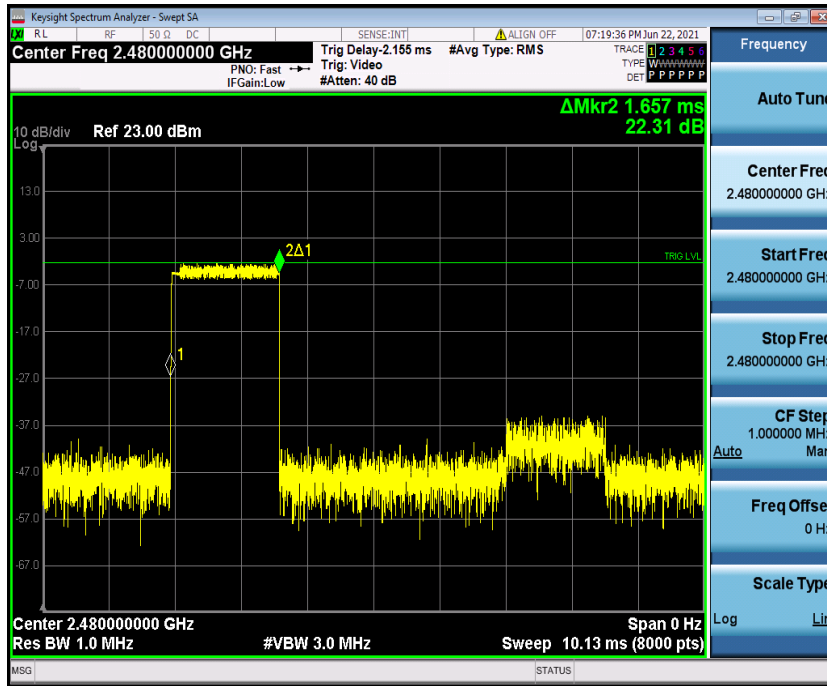
2DH3_Ant1_Hop_2480
