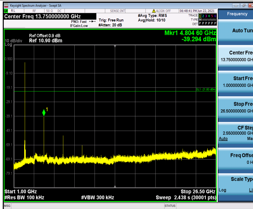
2DH5_Ant1_2402_1000~26500
