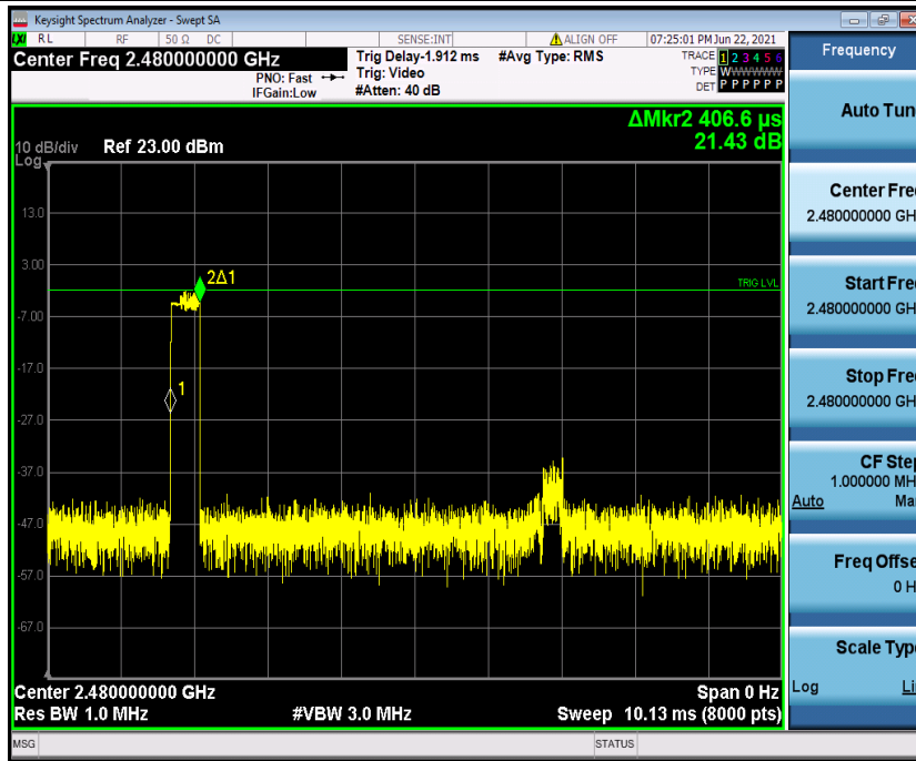
3DH1_Ant1_Hop_2480
