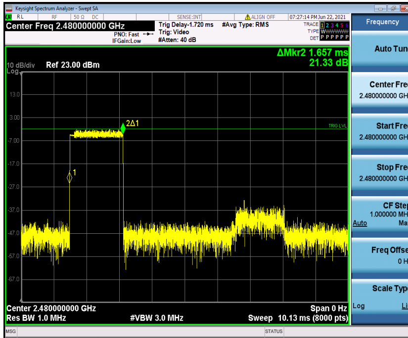
3DH3_Ant1_Hop_2480
