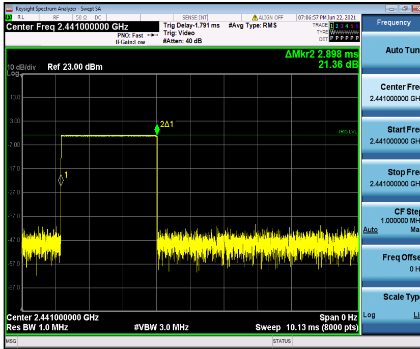
DH5_Ant1_Hop_2441
