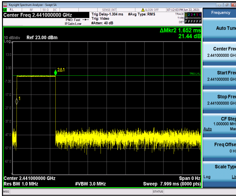
DH3_Ant1_Hop_2441
