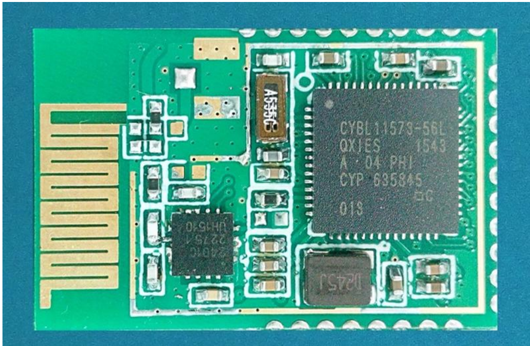
(4) EUT Photo
