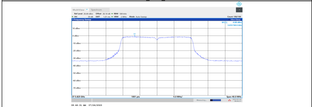
11A_Ant3_5825
