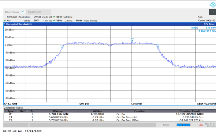
11N20SISO_Ant3_5700
