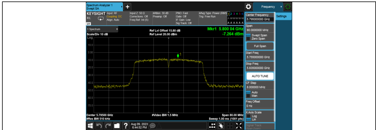
11N40MIMO_Ant1_5795
