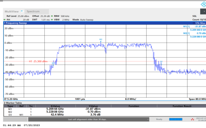
11N40SISO_Ant3_5230
