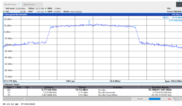
11AC80MIMO_Ant1_5775
