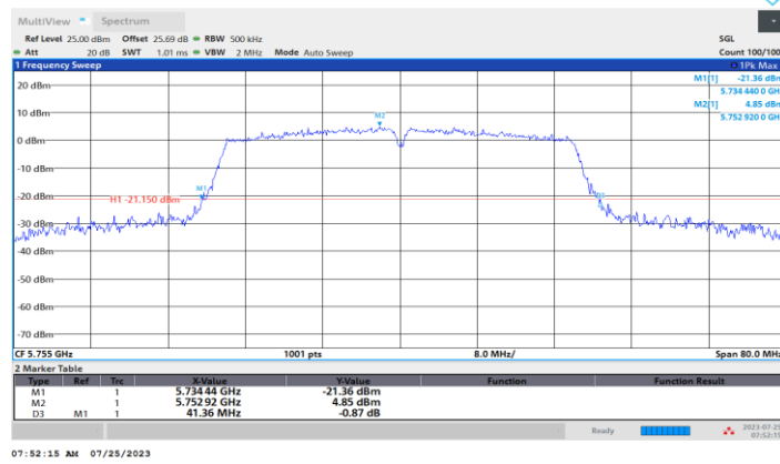
11N40MIMO_Ant1_5755
