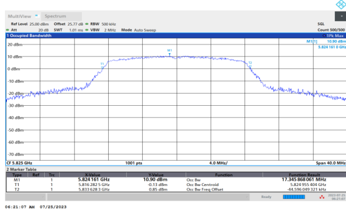
11A_Ant2_5825
