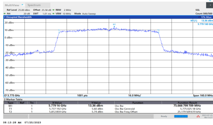
11AC80MIMO_Ant2_5775
