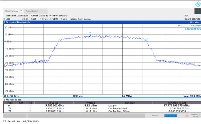
11N20MIMO_Ant2_5785
