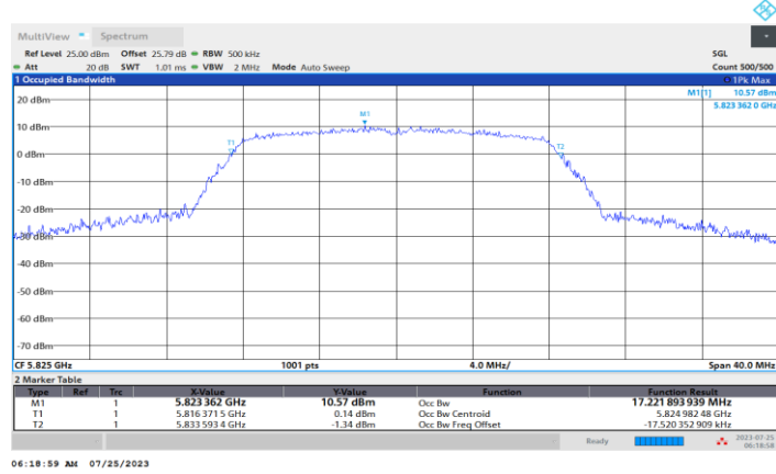
11A_Ant1_5825
