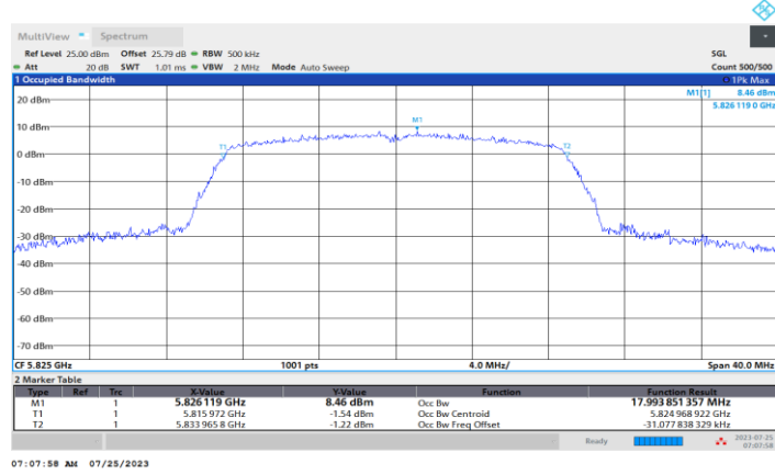
11N20MIMO_Ant1_5825
