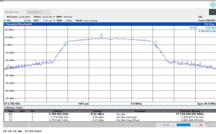
11A_Ant2_5785
