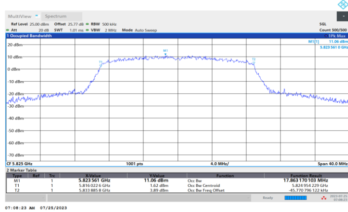
11N20MIMO_Ant2_5825
