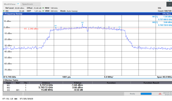
11N20MIMO_Ant2_5745
