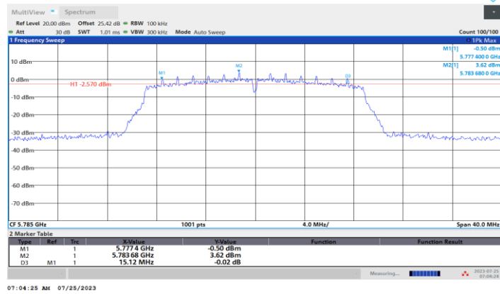
11N20MIMO_Ant1_5785
