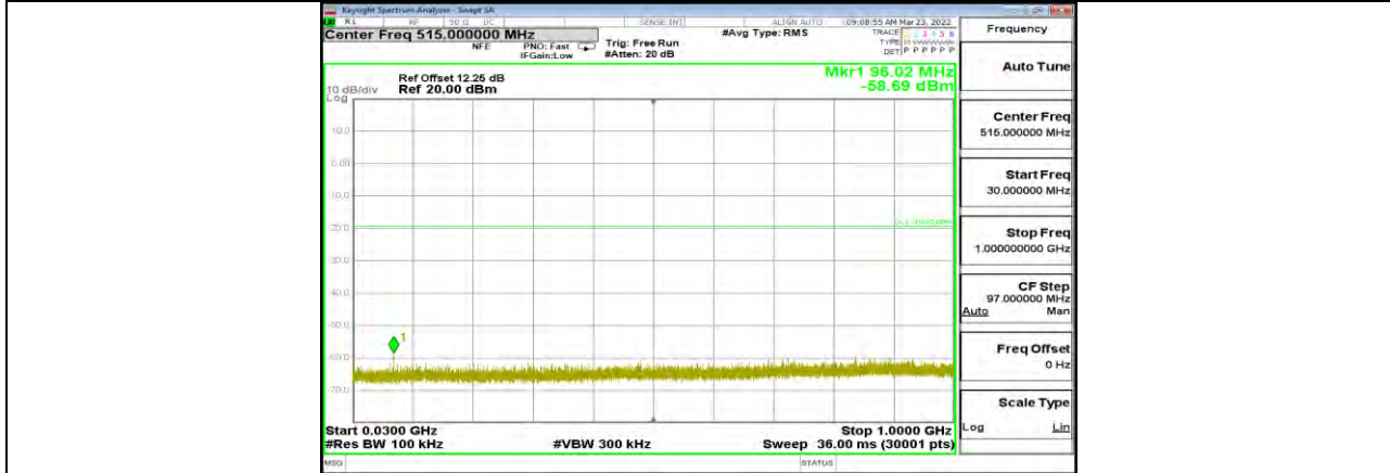
2DH5 Ant1 2441 30~1000
