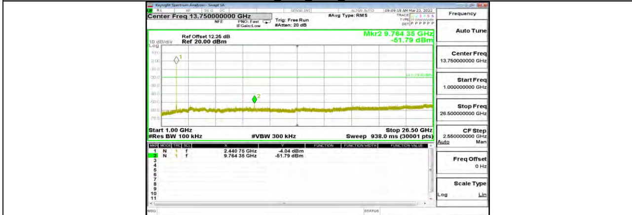
2DH5 Ant1 2441 1000~26500
