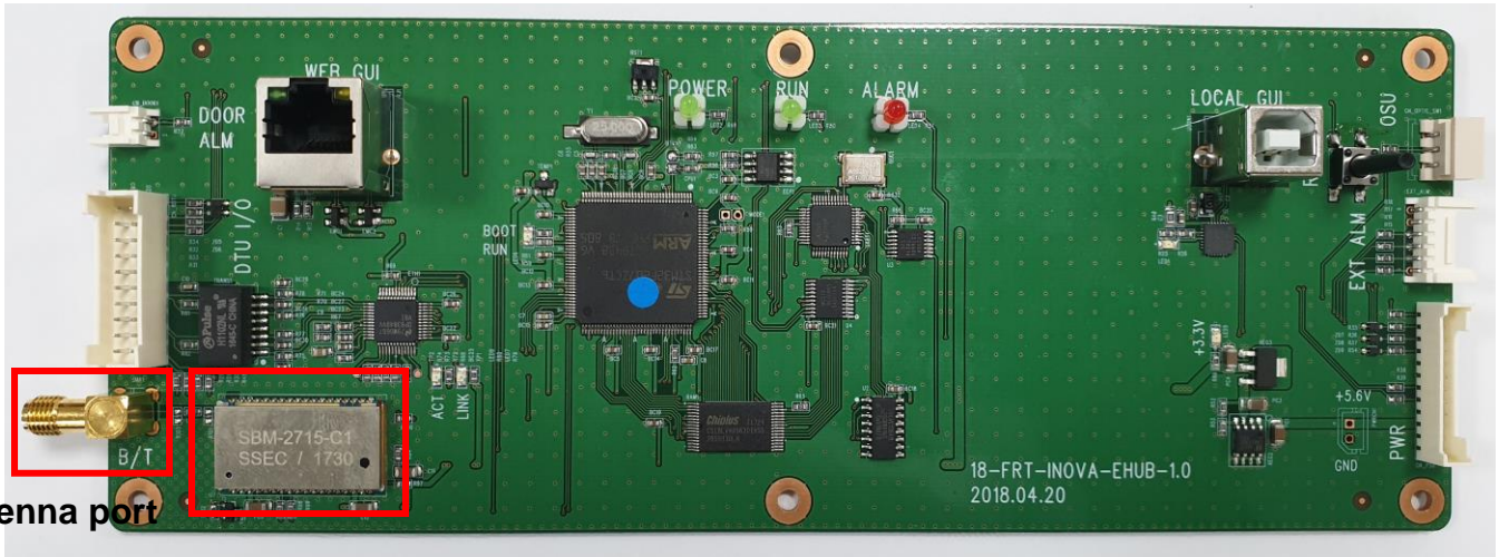
BT Module
