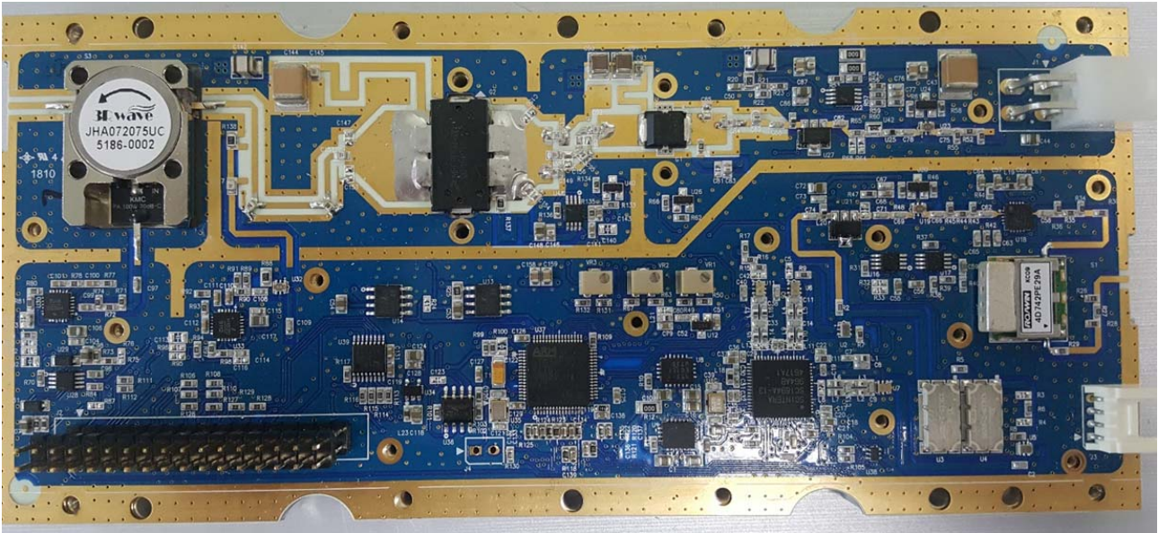
_PCB Top_TX
