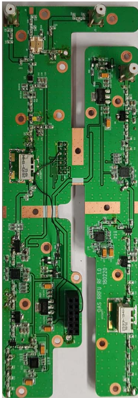
_PCB Top_RF
