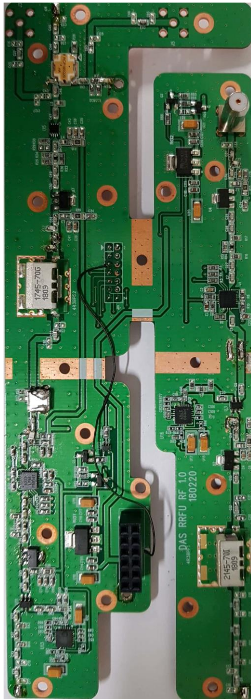
_PCB Top_RF
