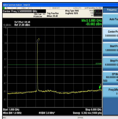
Band41-10MHz-QPSK-40620-50RB#0-Range2:1000~6000MHz
