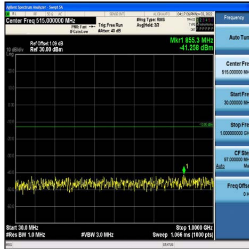
Band4-1.4MHz-QPSK-20393-6RB#0-Range1:30~1000MHz
