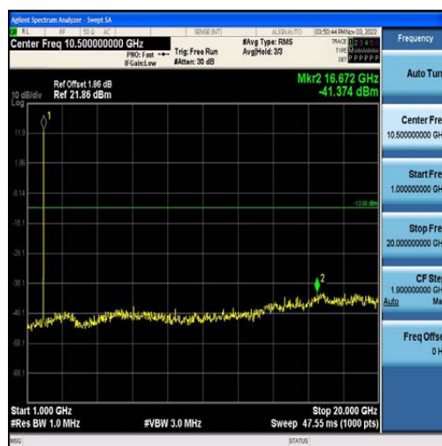
Band2-10MHz-QPSK-19150-50RB#0-Range2:1000~20000MHz
