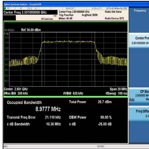
Band41-10MHz-QPSK-39700-50RB#0-8.9777
