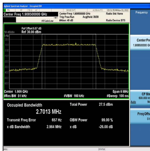
Band2-3MHz-QPSK-19185-15RB#0-2.7013
