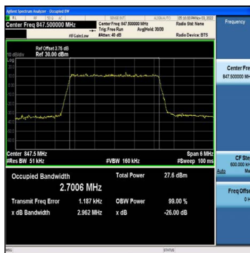
Band5-3MHz-QPSK-20635-15RB#0-2.7006
