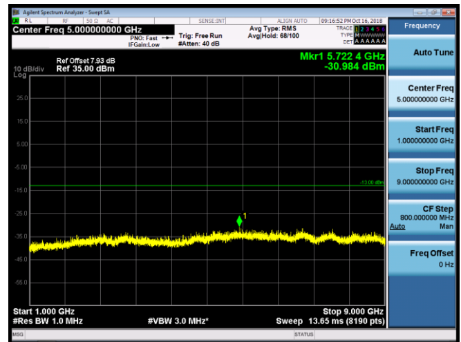
GSM 850-MCH-GSM
