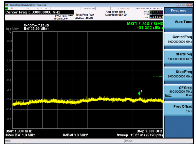
GSM 850-LCH-GSM
