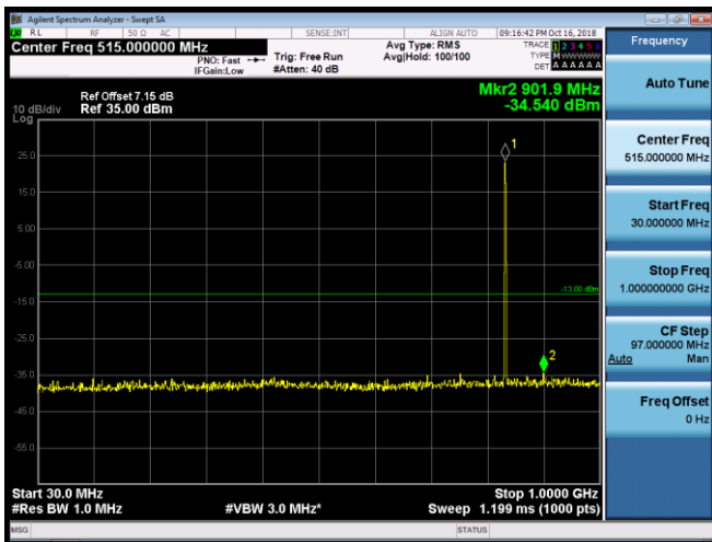
GSM 850-MCH-GSM
