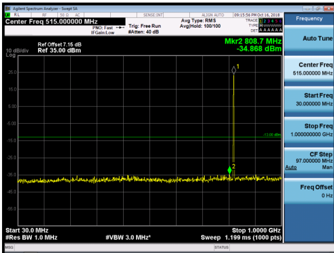
GSM 850-LCH-GSM
