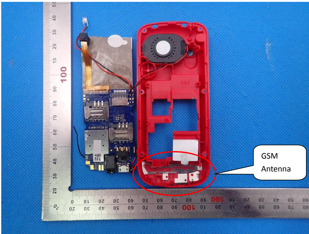
GSM ANTENNA
