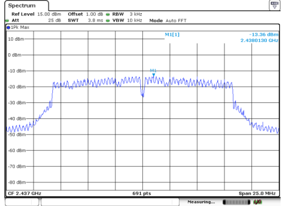
CH06
