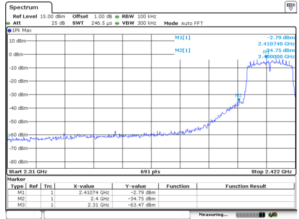
CH01-Bandedge
