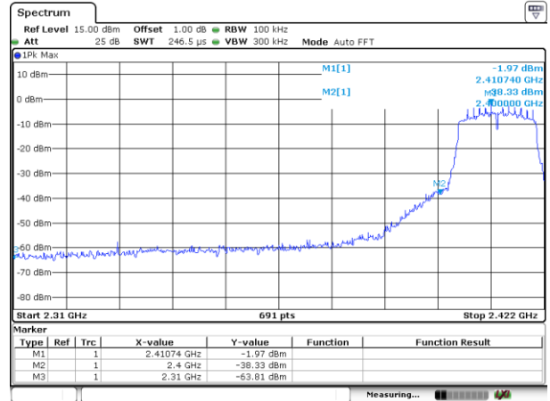
CH01-Bandedge
