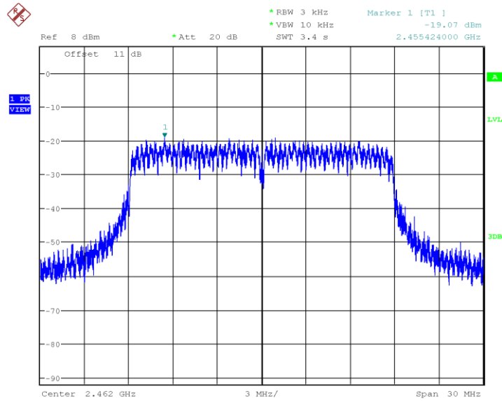
Plot 27. 802.11n HT20, 2462MHz PSD
