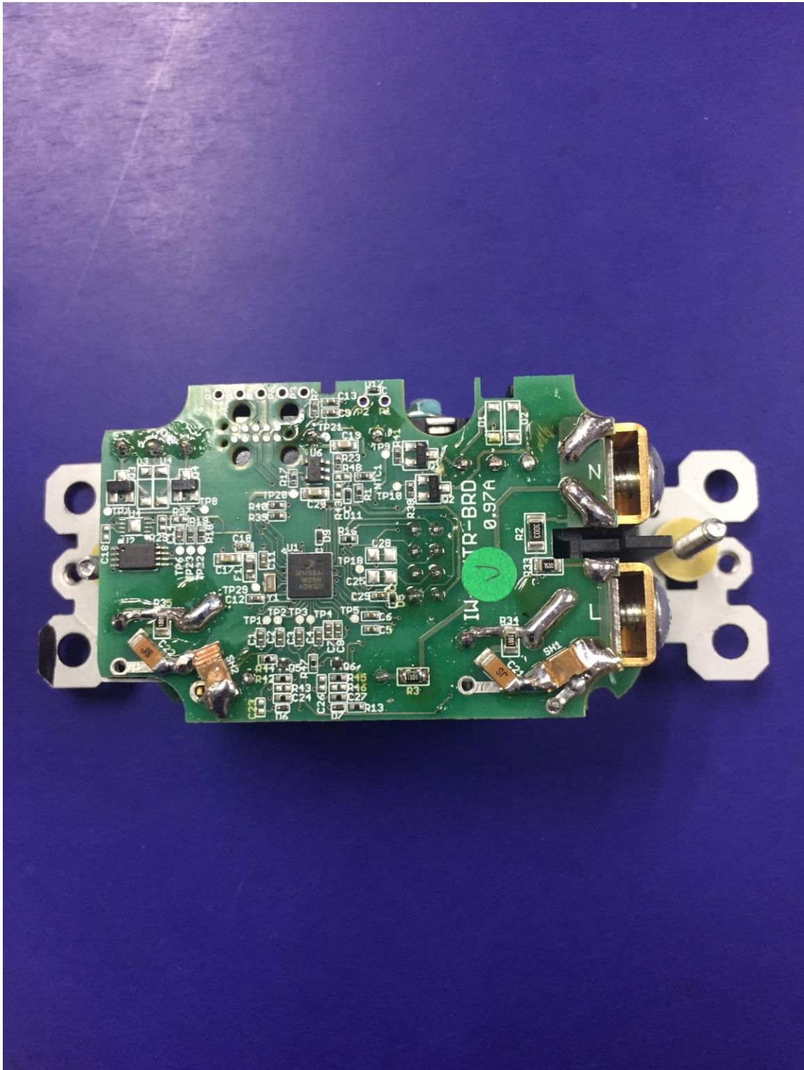
EUT Power PCB Bottom
