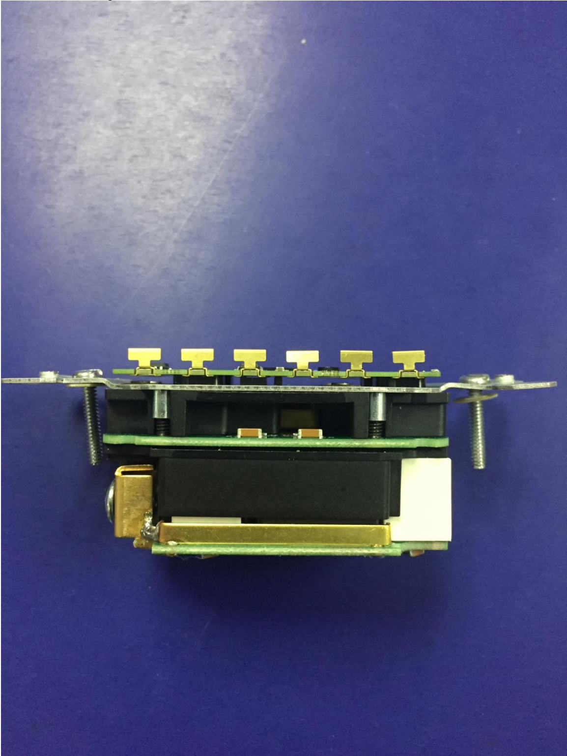
EUT RF PCB Right Side
