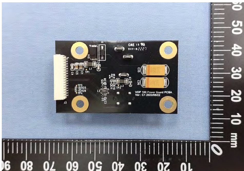
EUT Photo (52)
