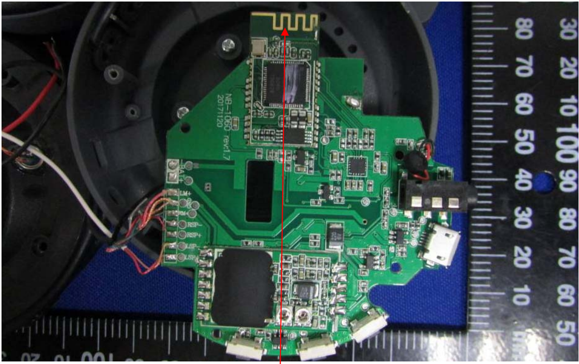
Antenna
