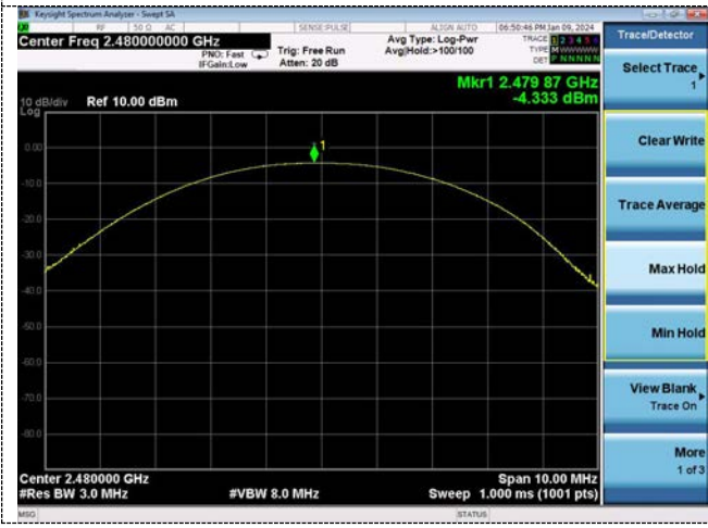
GFSK(CH78)
