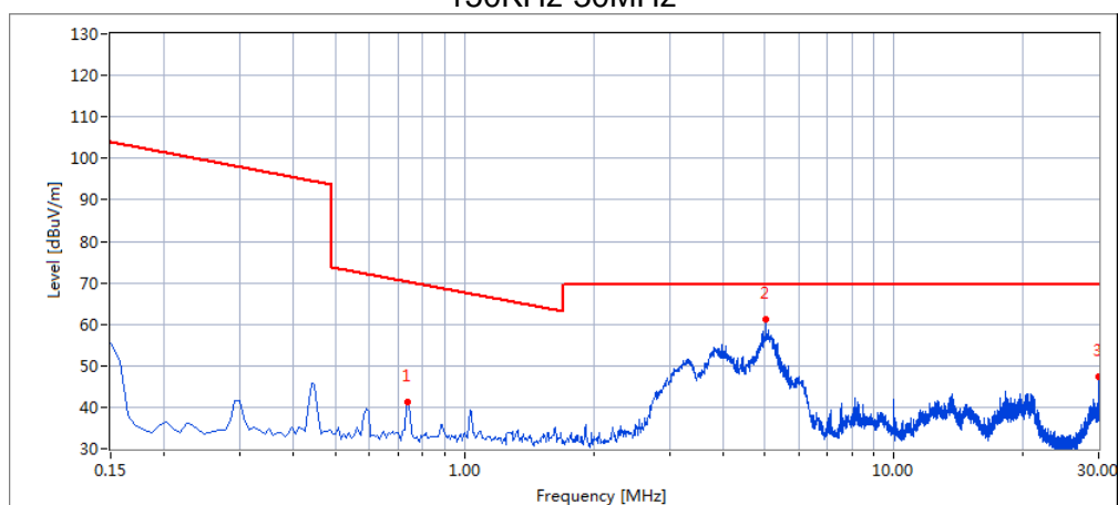
150KHz-30MHz
