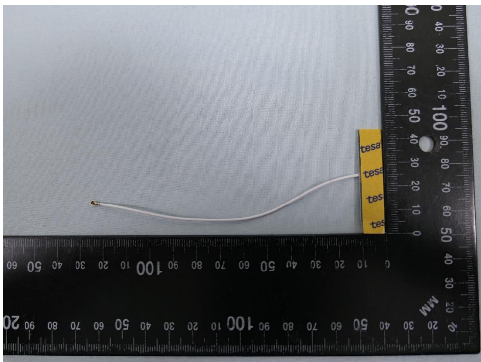
(12) PCB Antenna
