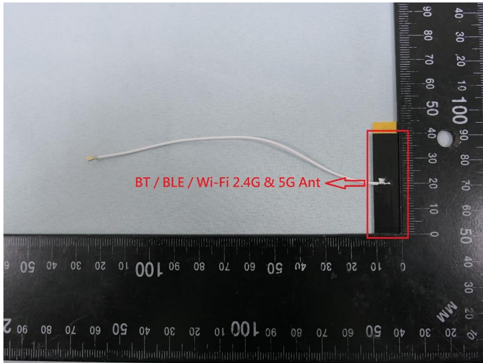
(12) PCB Antenna
