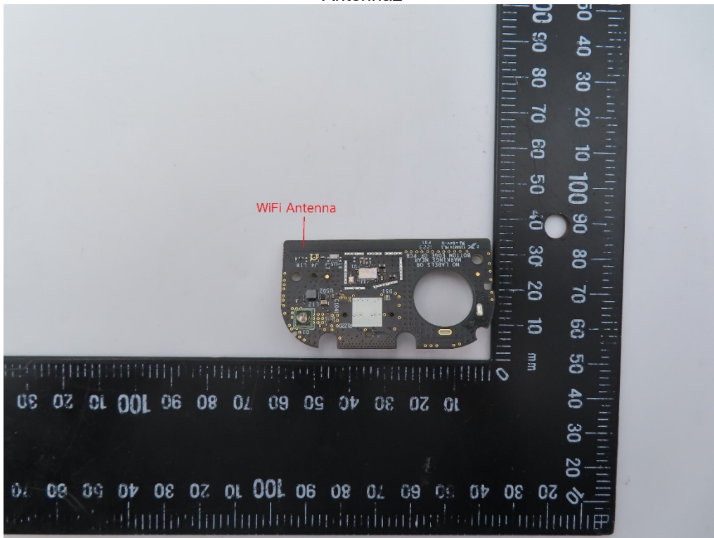
Antenna2
