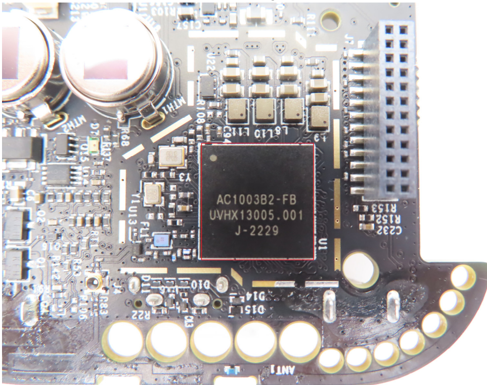
RF IC
