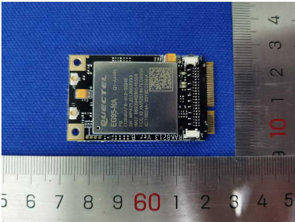
LTE module
