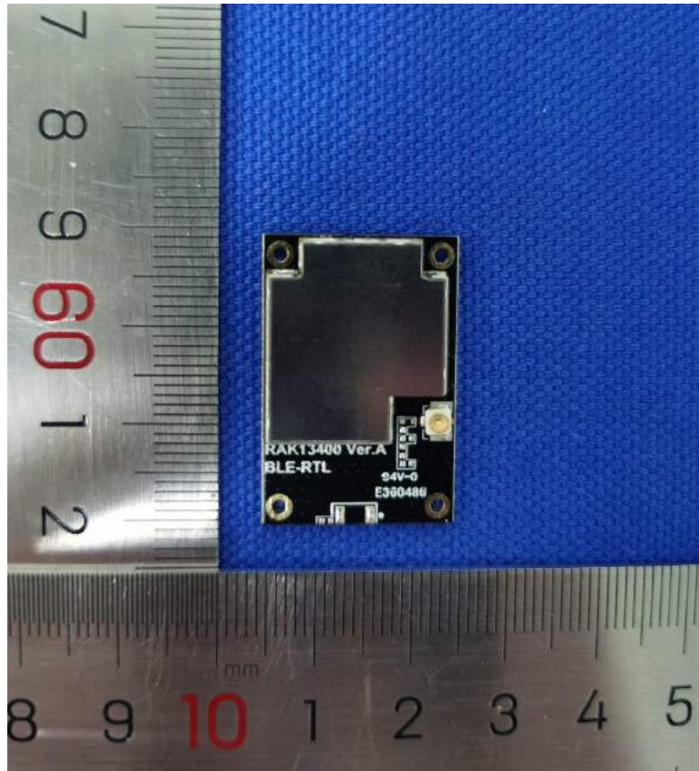
BLE module
