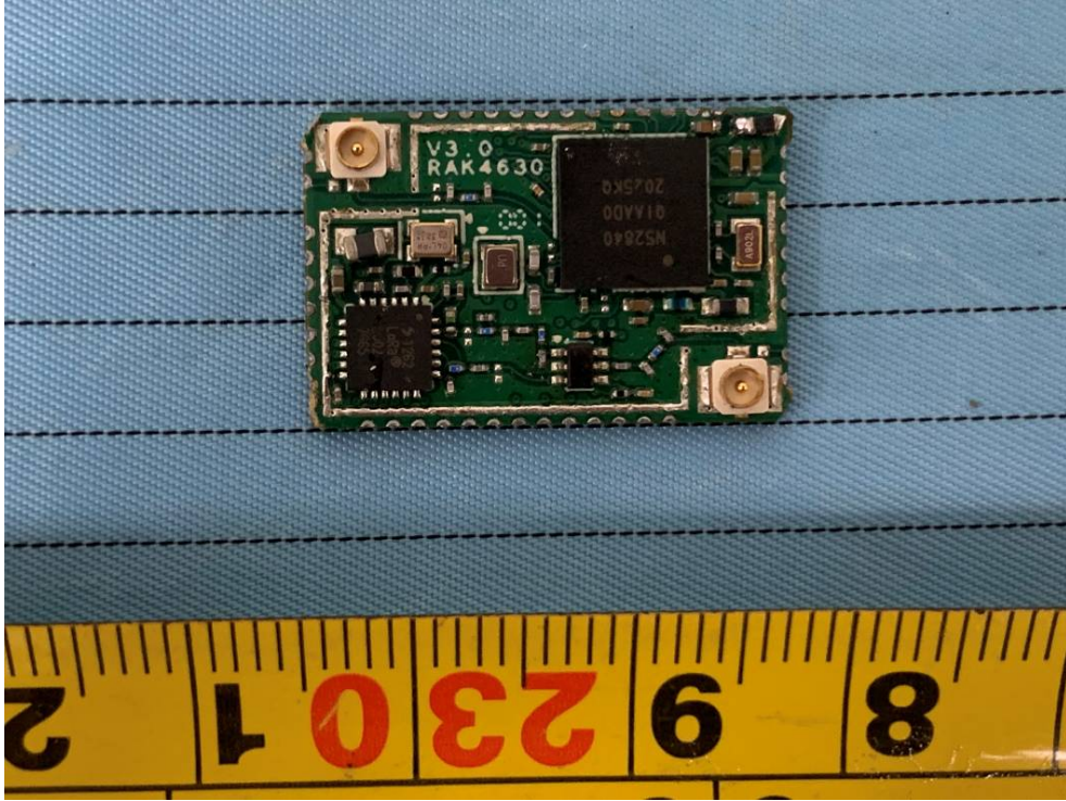
Model: RAK4630
